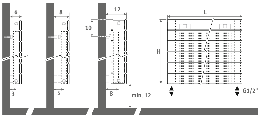
Typ 11 standardní stěnový úchyt
